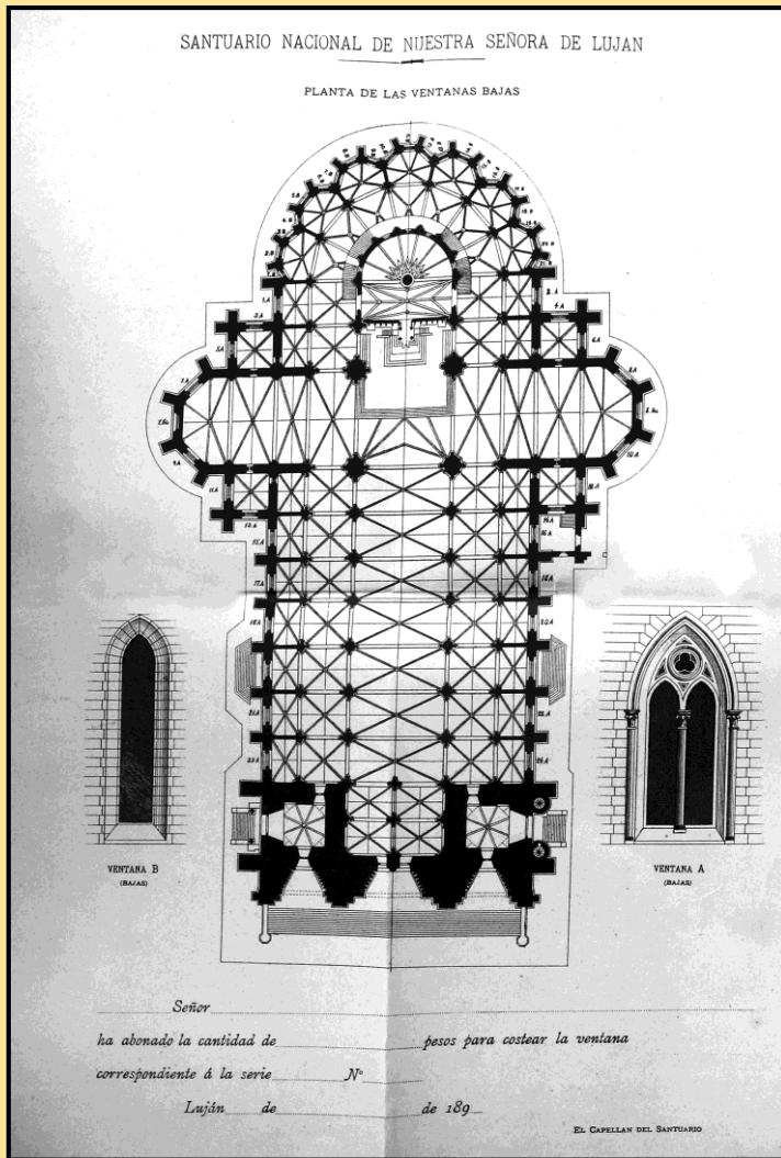
Plano de la planta de la futura Basílica.
